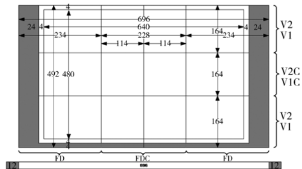
图 1 KAI-0340DM 结构示意图
